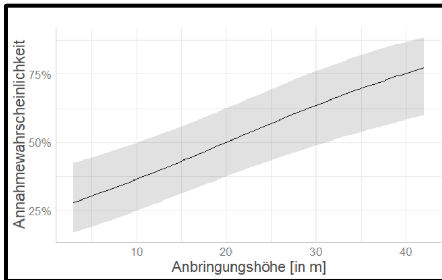
Abbildung 12: Annahmewahrscheinlichkeit einer Brutstätte durch Mehlschwalben in Abhängigkeit von der Anbringungshöhe. Logistische Regressionsanalyse des Parameters „Anbringungshöhe“ ( p \leq 0.001 , höchstsignifikant; ANOVA type III, Wald chisquare tests, n= 310 ).
