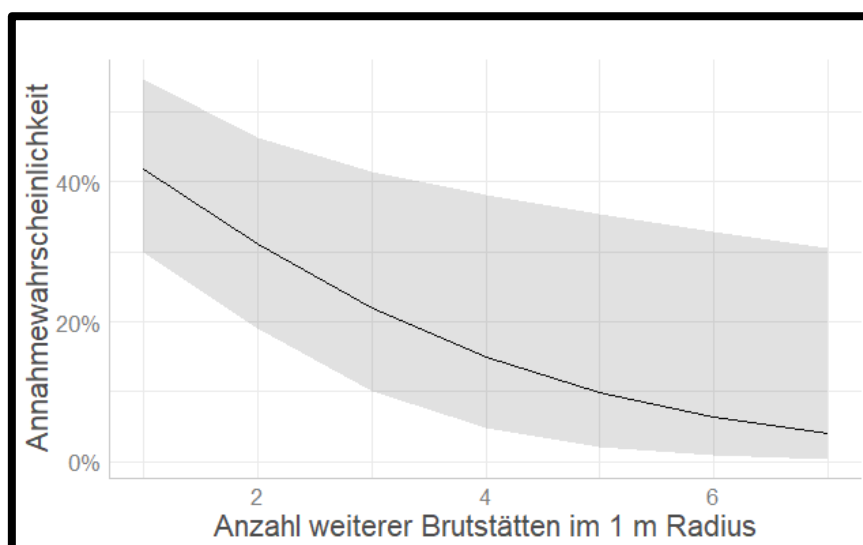
Abbildung 11: Annahmewahrscheinlichkeit einer Brutstätte durch Mehlschwalben in Abhängigkeit von der Anzahl weiterer Brutstätten in einem 1 Meter Radius. Logistische Regressionsanalyse des Parameters „Anzahl weiterer Brutstätten im 1 Meter Radius“ ( p \leq 0.01 , sehr signifikant; ANOVA type III, Wald chisquare tests, n= 310 )
