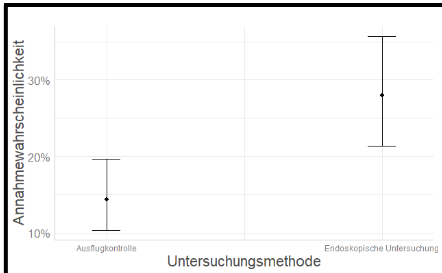
Abbildung 13: Annahmewahrscheinlichkeit eines Quartiers durch Fledermäuse in Abhängigkeit der Untersuchungsmethode (n= 372)
