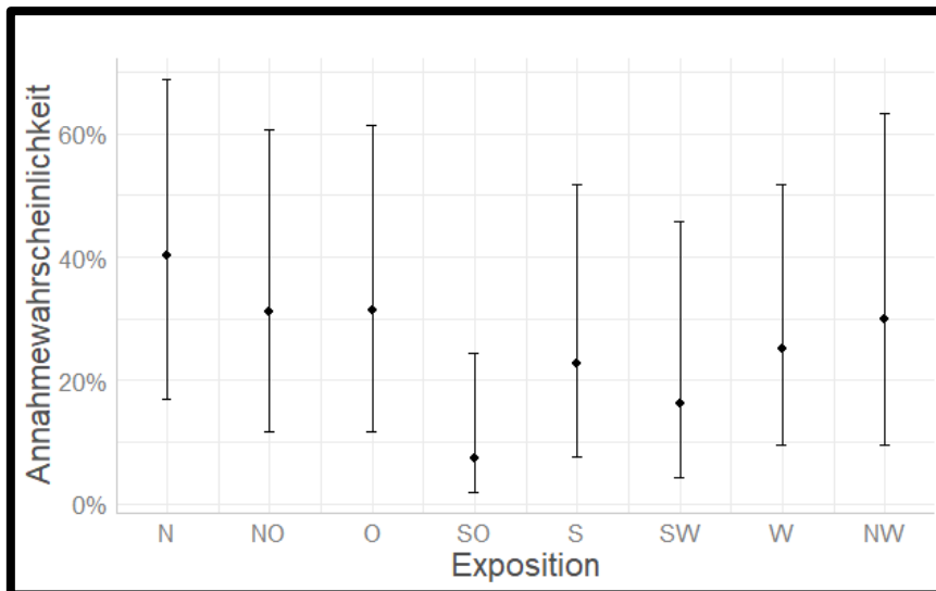
Abbildung 5: Annahmewahrscheinlichkeit einer Brutstätte durch Mauersegler in Abhängigkeit von der Exposition. Logistische Regressionsanalyse des Parameters „Exposition“ ( p \leq 0.001 , höchst signifikant; ANOVA type III, Wald chisquare tests, n= 869 )
