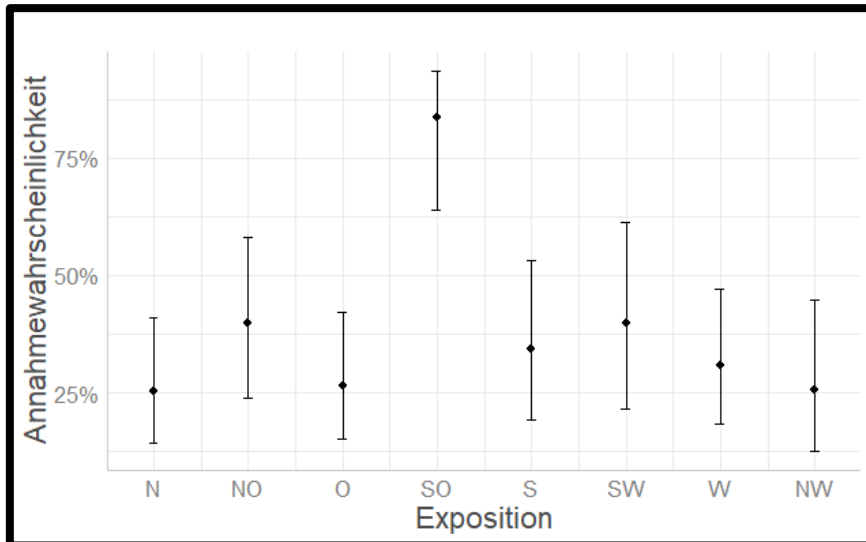
Abbildung 2: Annahmewahrscheinlichkeit einer Brutstätte durch Haussperlinge in Abhängigkeit von der Exposition. Logistische Regressionsanalysen des Parameters „Exposition“ ( p \leq 0.001 , höchst signifikant; ANOVA type III, Wald chisquare tests, n = 1.498 )
