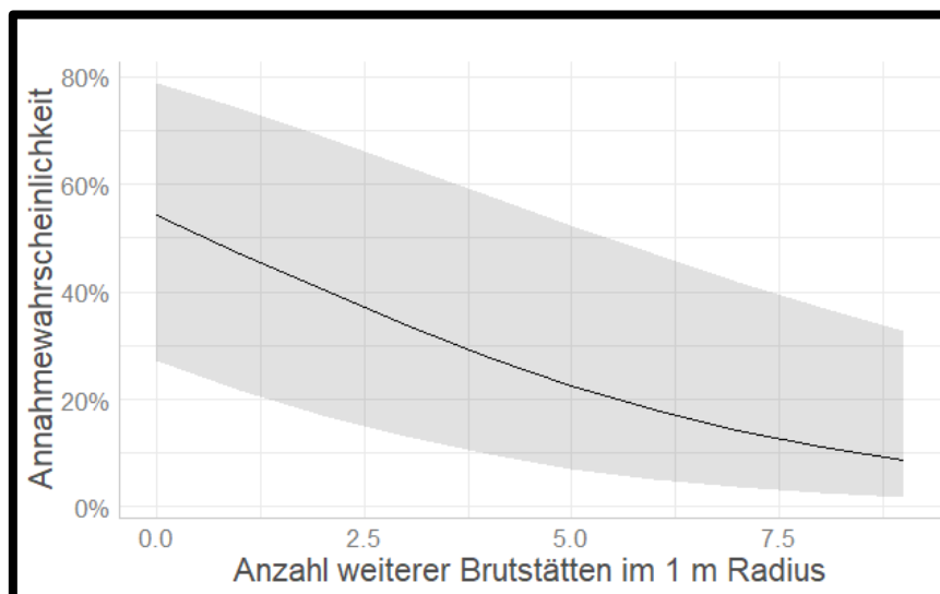
Abbildung 6: Annahmewahrscheinlichkeit einer Brutstätte durch Mauersegler in Abhängigkeit der Anzahl der Brutstätten im 1 Meter Radius um das Einflugloch. Logistische Regressionsanalyse des Parameters „Anzahl weiterer Brutstätten im 1 Meter Radius“ ( p \leq 0.001 , höchst signifikant; ANOVA type III, Wald chisquare tests, n= 869 )
