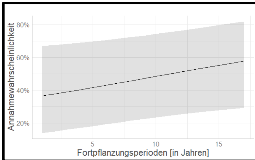
Abbildung 7: Annahmewahrscheinlichkeit einer Brutstätte durch Mauersegler in Abhängigkeit vom Alter. Logistische Regressionsanalyse des Parameters „Fortpflanzungsperioden in Jahren“ ( p > 0.05 ; p = 0.06 ; tendenziell signifikant; ANOVA type III, Wald chisquare tests, n = 869 )
