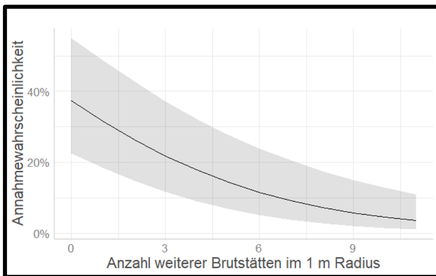
Abbildung 3: Annahmewahrscheinlichkeit einer Brutstätte durch Haussperlinge in Abhängigkeit der Anzahl weiterer Brutstätten im 1 m Radius um das Einflugloch. Logistische Regressionsanalyse des Parameters „Anzahl weiterer Brutstätten im 1 m Radius“ ( p \leq 0.001 , höchst signifikant; ANOVA type III, Wald chisquare tests, n = 1.498 )
