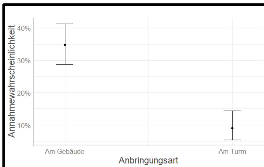
Abbildung 9: Annahmewahrscheinlichkeit einer Brutstätte durch Mehlschwalben in Abhängigkeit der Anbringungsart am Gebäude oder am Schwalbenturm (n= 728)
