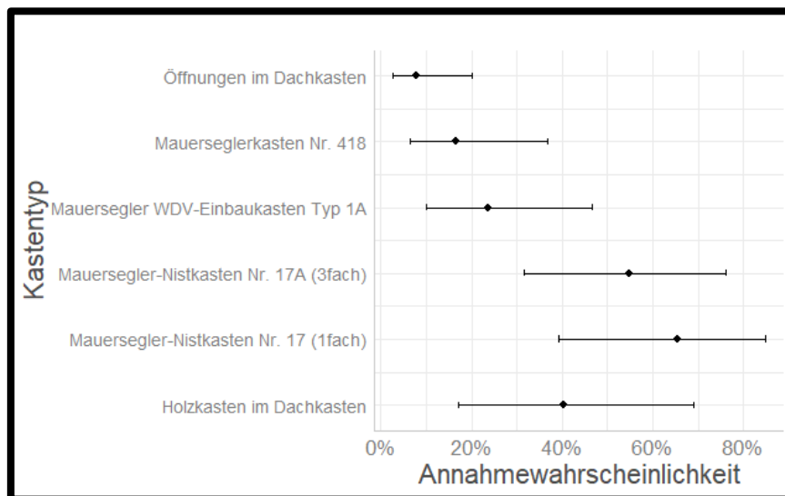
Abbildung 4: Annahmewahrscheinlichkeit einer Brutstätte durch Mauersegler in Abhängigkeit vom Brutstättentyp/Kastentyp. Logistische Regressionsanalyse des Parameters „Kastentyp“ ( p \leq 0.001 , höchst signifikant; ANOVA type III, Wald chisquare tests, n = 869 )
