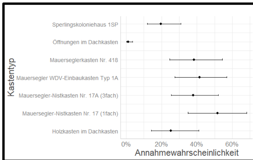
Abbildung 1: Annahmewahrscheinlichkeit einer Brutstätte durch Haussperlinge in Abhängigkeit vom Brutstättentyp/Kastentyp. Logistische Regressionsanalyse des Parameters „Kastentyp“ ( p \leq 0.001 , höchst signifikant; ANOVA type III, Wald chisquare tests, n = 1.498 )
