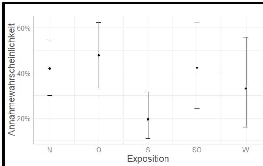
Abbildung 10: Annahmewahrscheinlichkeit einer Brutstätte durch Mehlschwalben in Abhängigkeit von der Exposition. Logistische Regressionsanalyse des Parameters „Exposition“ ( p \leq 0.01 , sehr signifikant; ANOVA type III, Wald chisquare tests, n= 310 )
