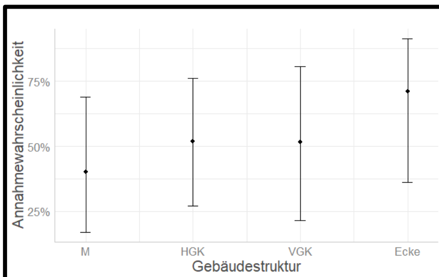
Abbildung 8: Annahmewahrscheinlichkeit einer Brutstätte durch Mauersegler in Abhängigkeit von der Gebäudestruktur. Logistische Regressionsanalyse des Parameters „Gebäudestruktur“ ( p > 0.05 ; p = 0.09 ; tendenziell signifikant; ANOVA type III, Wald chisquare tests, n = 869 ); M = Fassadenmitte, HGK = horizontale Gebäudekante, VGK = vertikale Gebäudekante, Ecke = nahe Dachecke
